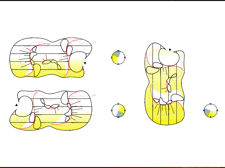
Belichtungskonzept Morgens viel Sonneneinfall, Mittags keinen und Abends geringen
